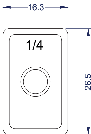
Vista Planta
